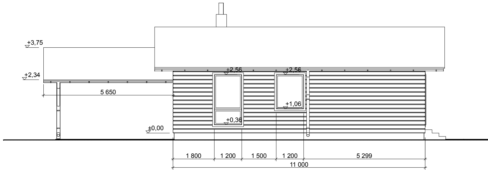
Fasāde A-2
